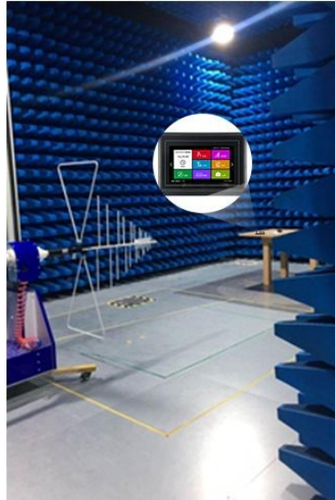
图 5-4 RE 测试图
