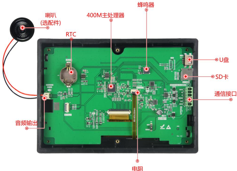
图 1-2 硬件配置图
